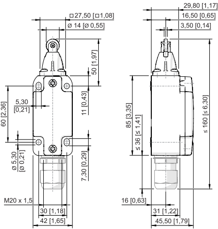
Rollenstößel 8070/2--R-U60
