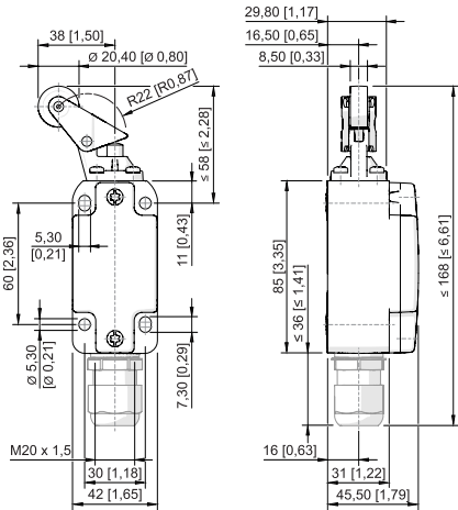
Rollenhebel 8070/2-.-WPH-U60
