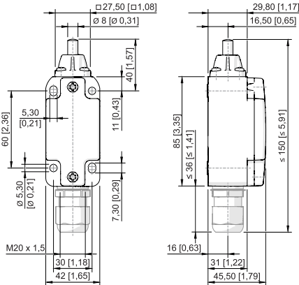
Kuppenstoßel 8070/2-3-W-U60
