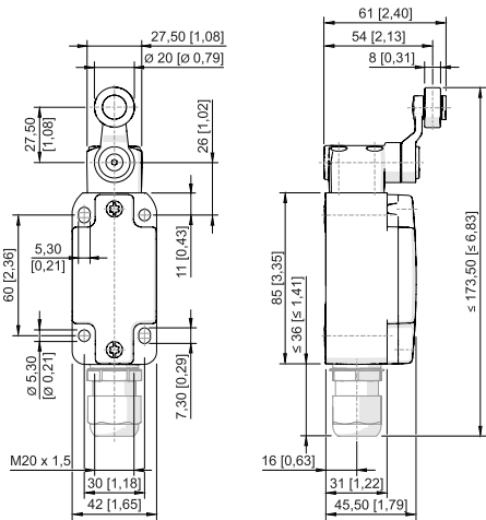
Schwenkhebel 8070/2-D-U60
