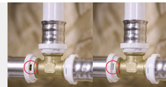
Visuele inspectie. Juiste insteekdiepte wordt bereikt als de buis de inspectievensters volledig afdekt of wit kleurt.
