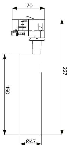
LEDspot3C-C-CS 10W
