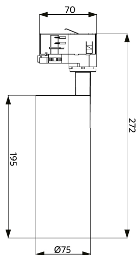
LEDspot3C-C-CS 30W
