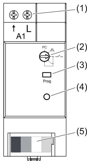
Bild 1: Geräteaufbau
