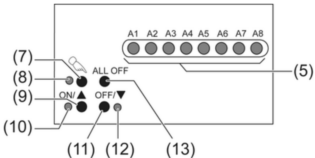
Bild 2: Bedienelemente – Übersicht
