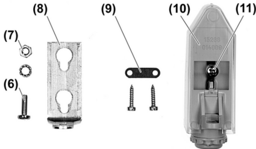
Bild 2: Sonnensensor und beiliegendes Zubehör
