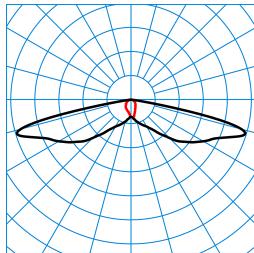
Publisca P3-SB3L-LR/1800-740 2G1 ET (CLO end value) TX300581
