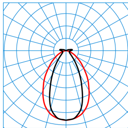
AragFHE 15 PN 100-840 ET PC LHT TX782601
