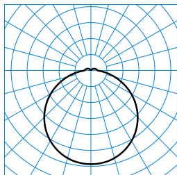
Olisq RWD1 DW 10-840 ETBLE +CAS IP54 + Olisq RWD1 C 01 TX565910
