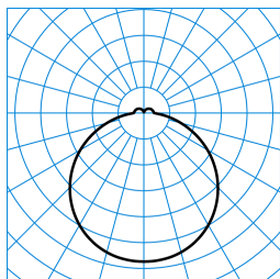
Olisq RWD1 DW 10-840 ETBLE +CAS IP54 + Olisq RWD1 ZDR 1/2 01 TX565914
