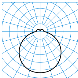
Olisq RWD1 DW 10-840 ETBLE +CAS IP54 TX565909
