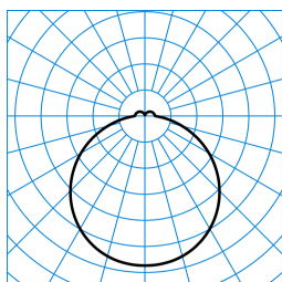
Olisq RWD1 DW 10-840 ETBLE +CAS IP54 + Olisq RWD1 ZDR 1/2 05 TX565916
