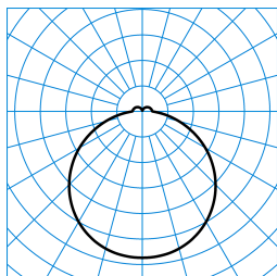
Olisq RWD1 DW 10-840 ETBLE +CAS IP54 + Olisq RWD1 ZDR 1/2 03 TX565915
