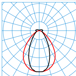
Tugra 15 PN 60-840 ETDD LLWC PC LV 23 TX777925
