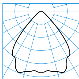
InperiaLP C05 HR22 1800-840 01 + RD-PC TX041213
