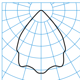
InperlaLP C05 HR22 1800-840 01 + ZN-PC ■ C0 - C180 TX041704
