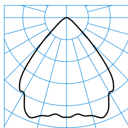
InperiaLP C05 HR22 1800-840 01 + DA 01 TX041209
