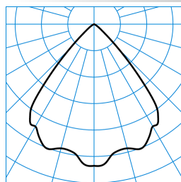
InperiaLP C05 HR22 1800-840 ET 01 TX768593
