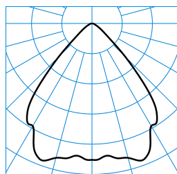
InperiaLP C05 HR22 1800-840 01 + DA 03 TX041210
