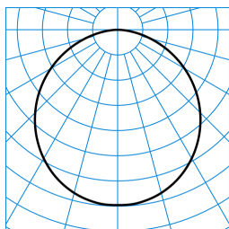
Olisq RWD2 DW 20-830 ETBLE +DMM IP54 + Olisq RWD2 ZDR 1/1 01 TX425900
