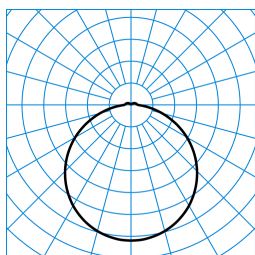
Olisq RWD2 DW 20-830 ETBLE +DMM IP54 + Olisq RWD2 C 01 TX425764
