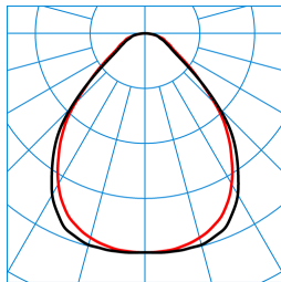
ArimoFit G2 M52 PW 20-830 ET TWW TX376407
