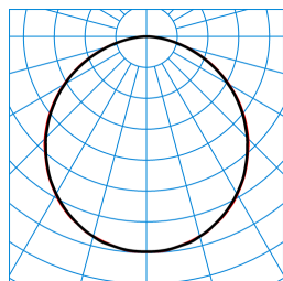
Olisq QWD3 DW 45-840 ET HFS IP54 + Olisq QWD3 ZDR 1/1 03 TX461379
