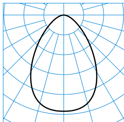
InperiaL G2 C07 BR19 1000-830 01 + DA-M 01 ■ C0 - C180 TX052552
