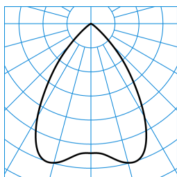
InperiaL G2 C07 BR19 1000-830 01 + DA 01 ■ C0 - C180 TX052551
