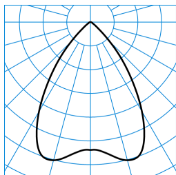
InperiaL G2 C07 BR19 1000-830 01 + RD-PC ■ C0 - C180 TX052553
