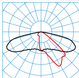
Cuvia 40-AB2L-LR/1650-740 2G1S ET TX778049
