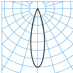
7651 LentyP L-MF 30-BF M54 ETBLE 01 (150) TX782073
