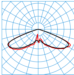
Publisca P2-RB6L/2000-730 3G1S TX047819
