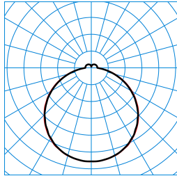
Olisq QWD2 DW 14-40/4/ML-830 IP54 IK ET (stage 1) TX777290
