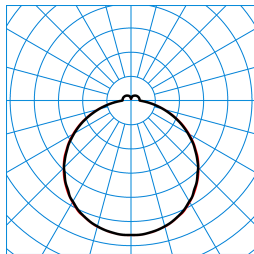
Olisq QWD2 DW 14-40/4/ML-830 IP54 IK ET (stage 3) TX777296
