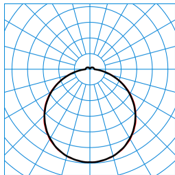
Olisq QWD2 DW 14-40/4/ML-830 IP54 IK ET + Olisq QWD2 ZDR 1/2 01 (stage 1) TX462357
