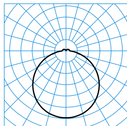
Olisq RWD3 DW 50-830 ET IP54 PC + Olisq RWD3 ZDR 1/2 05 TX429649
