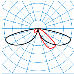
LTX PT-AB2L-LRA/15/18/26-740 4G1 (1500 lm) TX084150
