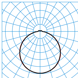
Olisq Act QWD2 DW 35 ETDD8 IP54 IK + Olisq QWD2 ZDR 1/2 01 (ACTDWW) TX462205
