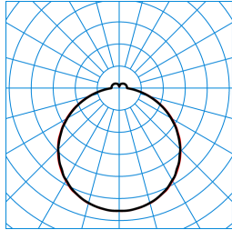
Olisq Act QWD2 DW 35 ETDD8 IP54 IK (ActDWW) TX777281
