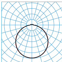
Olisq Act QWD2 DW 35 ETDD8 IP54 IK + Olisq QWD2 ZDR 1/2 03 (ACTDWW) TX460706
