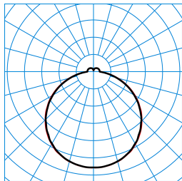
Olisq Act QWD2 DW 35 ETDD8 IP54 IK (ActDCW) TX777274
