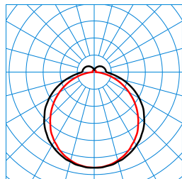
Olisq LWD3 DW 30-75/4/ML-830 ET IP54 IK (stage 2) TX564627
