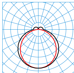
Olisq LWD3 DW 30-75/4/ML-830 ET IP54 IK (stage 4) TX564629
