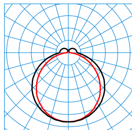
Olisq LWD3 DW 30-75/4/ML-830 ET IP54 IK (stage 3) TX564628
