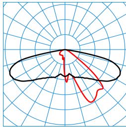
Publisca P2-AB2L/2000-740 3G1S TX047709
