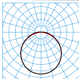
3331 G2 D3 LED4900-830 ET 03 TX771345
