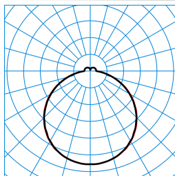
Olisq QWD2 DW 20-840 ET EB3 IP54 IK TX777364
