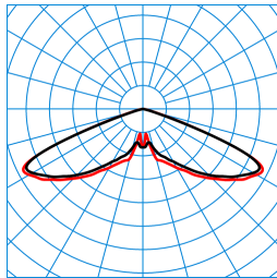
Publisca P1W-RB6L-LR/3200-740 4G1S ET (CLO initial value) TX300823
