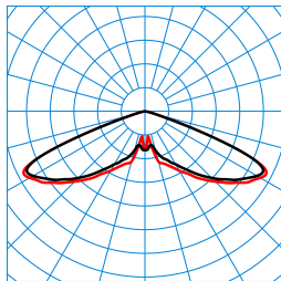
Publisca P1W-RB6L-LR/3200-740 4G1S ET (CLO end value) TX300550
