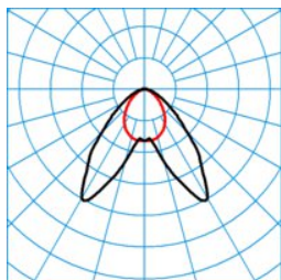
ELINE LDAH55-140 ML 840 L225 4 50
