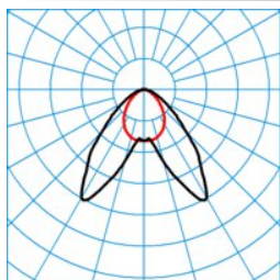
ELINE LDAH55-140 ML 840 L225 0 50
