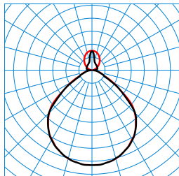
Luceos D/H1-L CDP 6700-840 ETDD 01 (Ceiling D1 ZD/01) TX547693
