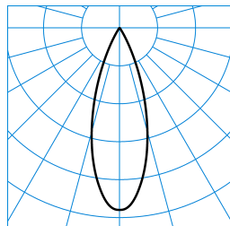
7651 Lentyp L-FL 30-827 M32 ET 05 (225) TX781788
