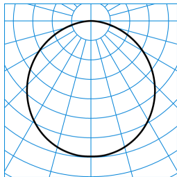
Olisq RWD2 DW 20-830 ET EB3 IP54 + Olisq RWD2 ZDR 1/1 01 TX425885
