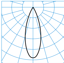
7651 Lentyp L-FL 40-827 M32 ET 05 (225) TX781793
