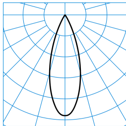
7651 Lentyp L-FL 40-827 M32 ET 05 (150) TX781791
