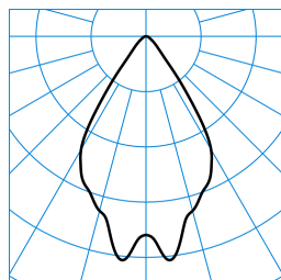
InperlaLP C05 BR22 2700-840 01 + RG-PC ■ C0 - C180 TX041575
