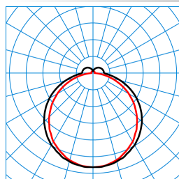
Olisq LWD2 DW 20-830 ET2 IK TX564806
