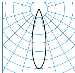
7651 Lentyp L-MF 40-830 M33 ETBLE 03 (225) TX782264
