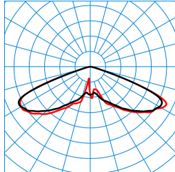
Publisca P2-RB6L-LRA/2000-730 3G1S TX047893
