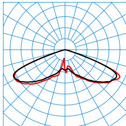
Publisca P2-RB6L-LRA/2000-730 3G1S ET (CLO initial value) TX301303
