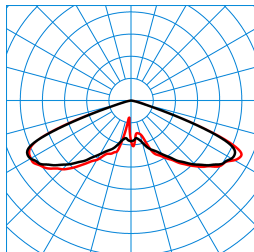
Publisca P2-RB6L-LRA/2000-730 3G1S ET (CLO end value) TX301385
