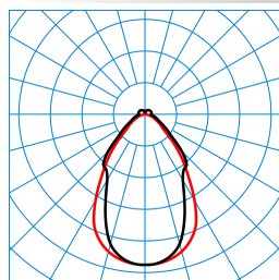
SFlow D2-L CDP-I 4300-840 ETDD UR 03 TX768925
