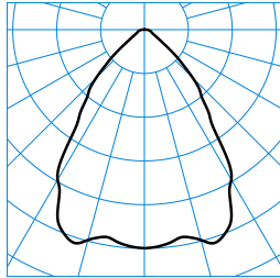
InperlaLP C05 BR25 2700-830 01 + ZN-PC ■ C0 - C180 TX041590
