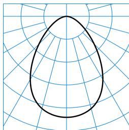
InperlaLP C05 BR25 2700-830 01 + DA-M 01 ■ C0 - C180 TX041586
