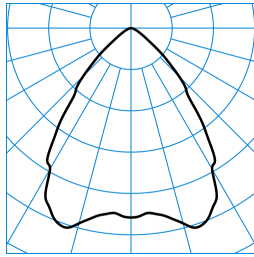
InperlaLP C05 BR25 2700-830 01 + RD-PC ■ C0 - C180 TX041588
