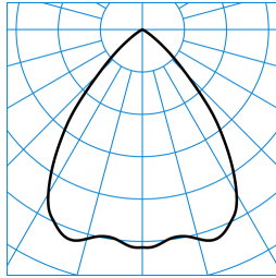
InperlaLP C05 BR25 2700-830 ETDD 01 ■ C0 - C180 TX771638
