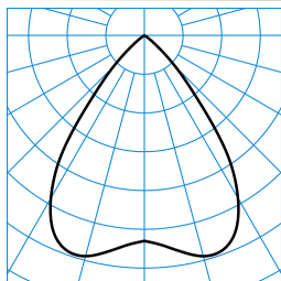
InperiaL G2 C07 BR19 2700-840 ETDD 03 ■ C0 - C180 TX768373
