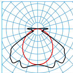
Nextrema G3 B 60-840 ET +LV TWP TX768561
