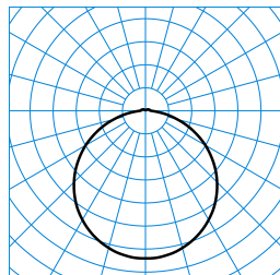
Olisq RWD4 DW 40-840 ETBLE +DMM IP54 PC + Olisq RWD4 C 01 TX375049
