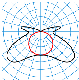
AragF 15 PXW 80-840 ETDD +LLWC LV PC TX782524
