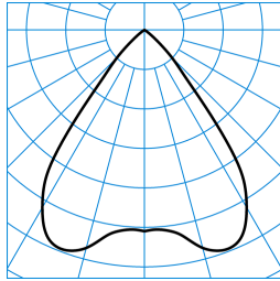
InperiaL G2 C07 HR19 1800-830 ETDD 03 ■ C0 - C180 TX769472
