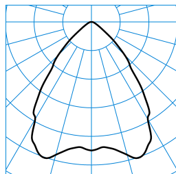
InperlaLP C05 BR22 1800-830 03 + RG-PC TX041241 ■ C0 - C180
