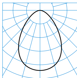
InperlaLP C05 BR22 1800-830 03 + DA-M 01 TX041548 ■ C0 - C180
