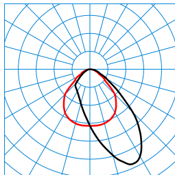
Luceos D/H2-L CDP-A 6500-830 01 (Ceiling D2 ZD/01) TX194609
