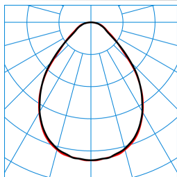
ArimoFit G2 D2 PW19 52-840 ETDD 01/01 TX376984
